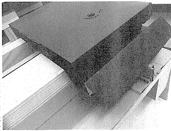
住宅で効果を発揮する立平用換気棟（片流れ）
