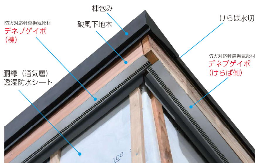
デネブゲイボ用部材 (別売)
