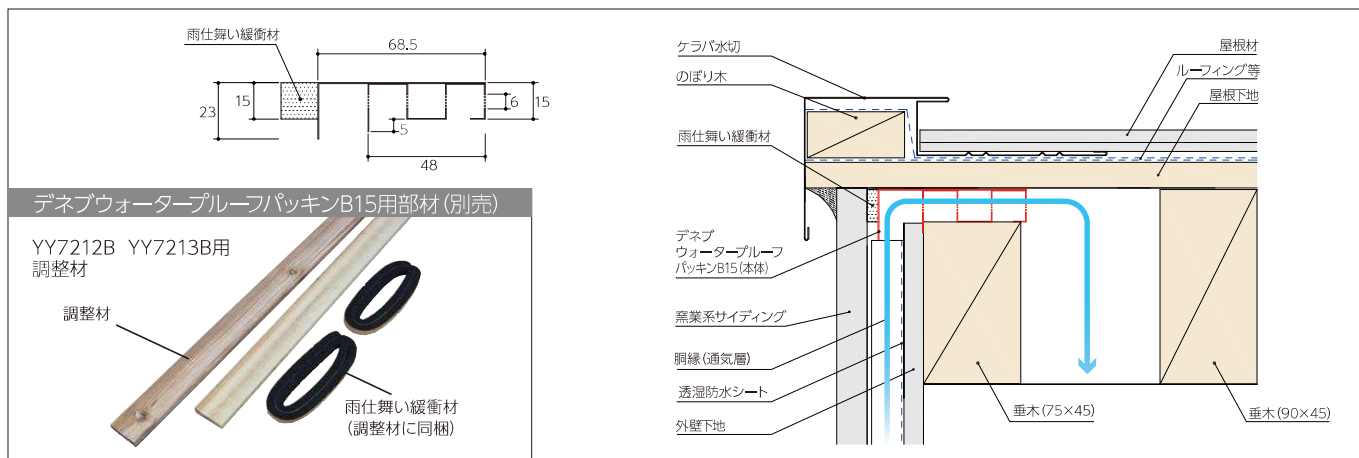
4. 野地板の取付
