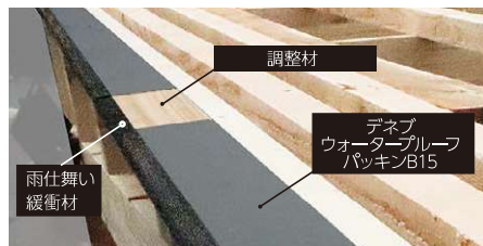
2. デネブウォータープルーフパッキンB15と調整材を取付
