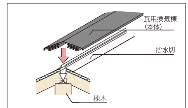
2. スピカKを取付け
