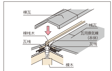
4. 棟瓦を取付ける
