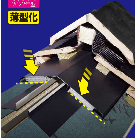
野地板を開口、捨て水切を取付けた状態
