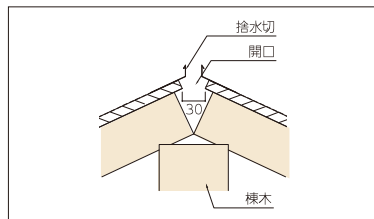
1. 野地板を開口、捨て水切を取付け
