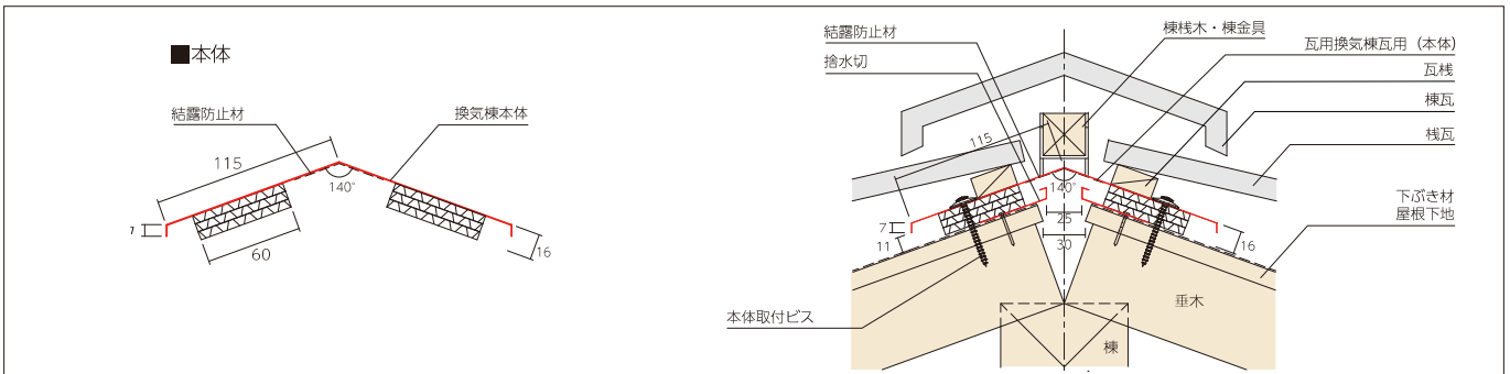
3. 棧瓦葺きを行う
