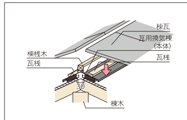
3. 棧瓦葺きを行う
